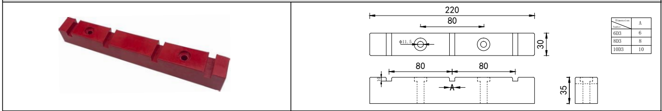
型号(mm) Item: 6D4 8D4 10D4系列 (80中心)
