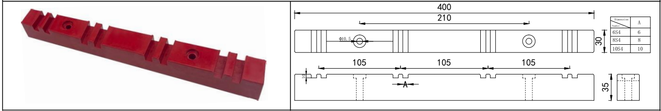
型号(mm) Item: 6D4 8D4 10D4系列 (105中心)
