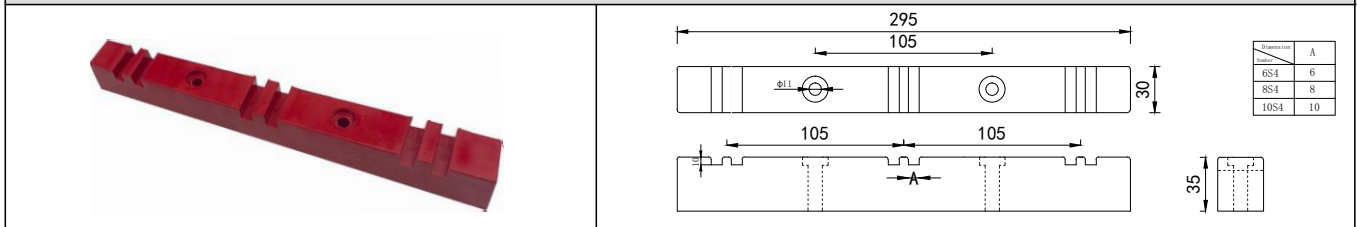
型号(mm) Item: 6S4B 8S4B 10S4B系列 (93中心)
