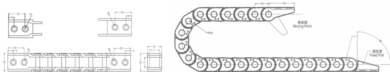
QSTL07 系列结构示意图
