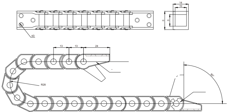
QSTL10 系列结构示意图
