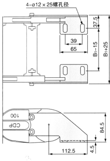
固定端/Fixed Bracket
