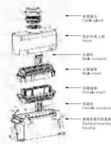
④ 表面安装，正面进线形式 Surface mounting and top entry type.
