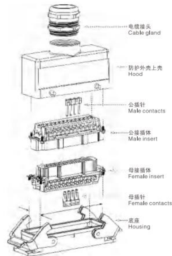
接插件安装示意图 Assembly details.
