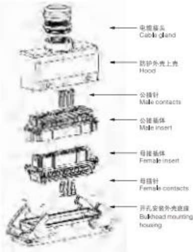
② 开孔安装，正面进线形式 Bulkhead mounting and top entry type.
