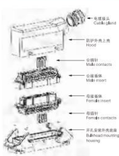
① 开孔安装，侧面进线形式 Bulkhead mounting and side entry type.
