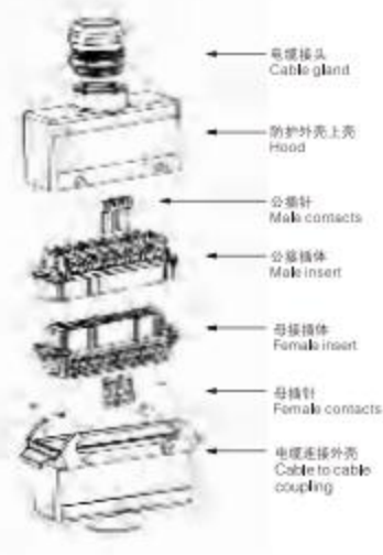
⑥ 电缆连接，正面进线形式 Cable to cable and top entry type.
