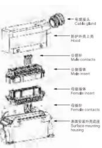
③ 表面安装，正面进线形式 Surface mounting and side entry type.
