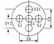
底部 BOTTOM
