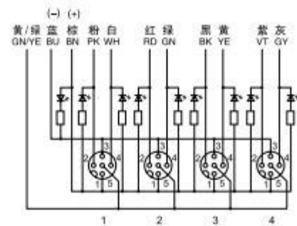
双通道 2 signals per port NPN
