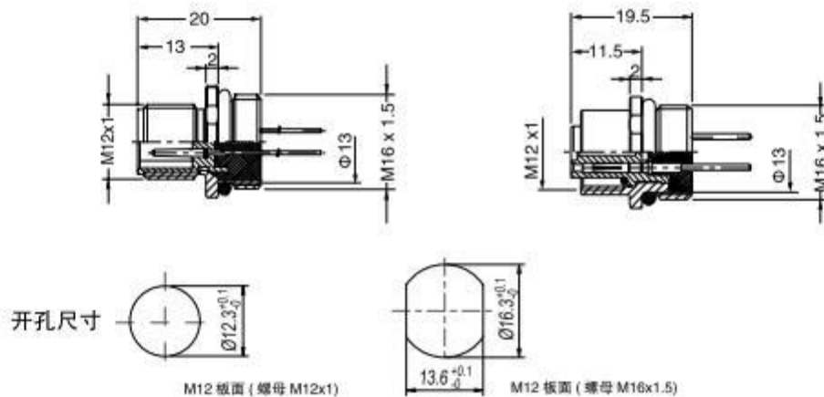
尺寸图 Description
