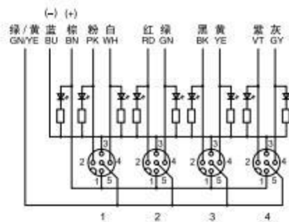
双通道 2 signals per port PNP
