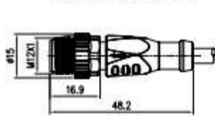
插针 Male 直出 Straight
