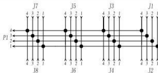
8 端口电路图
